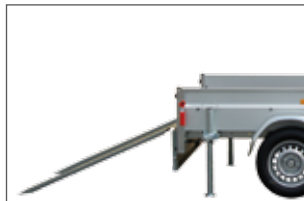
Abstellstützen & Auffahrschienen
