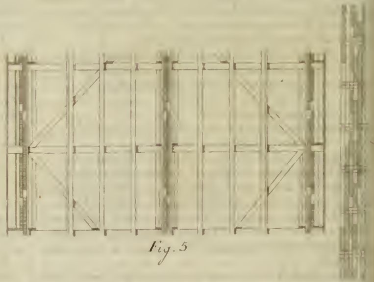
(Tavola complessiva del dettaglio per la costruzione de' ponti di legno)
