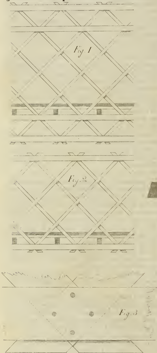
(Tavola complessiva del dettaglio per la costruzione de' ponti di legno)
